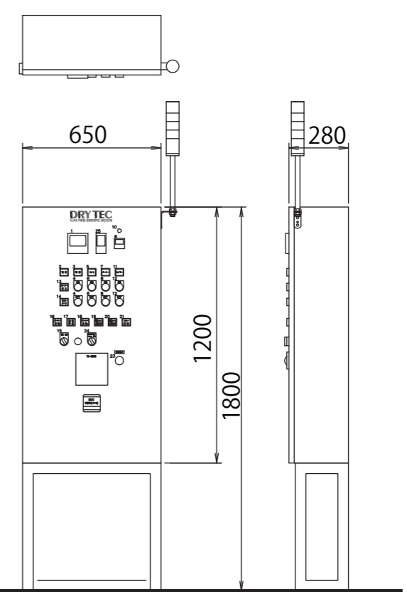
制御盤寸法
